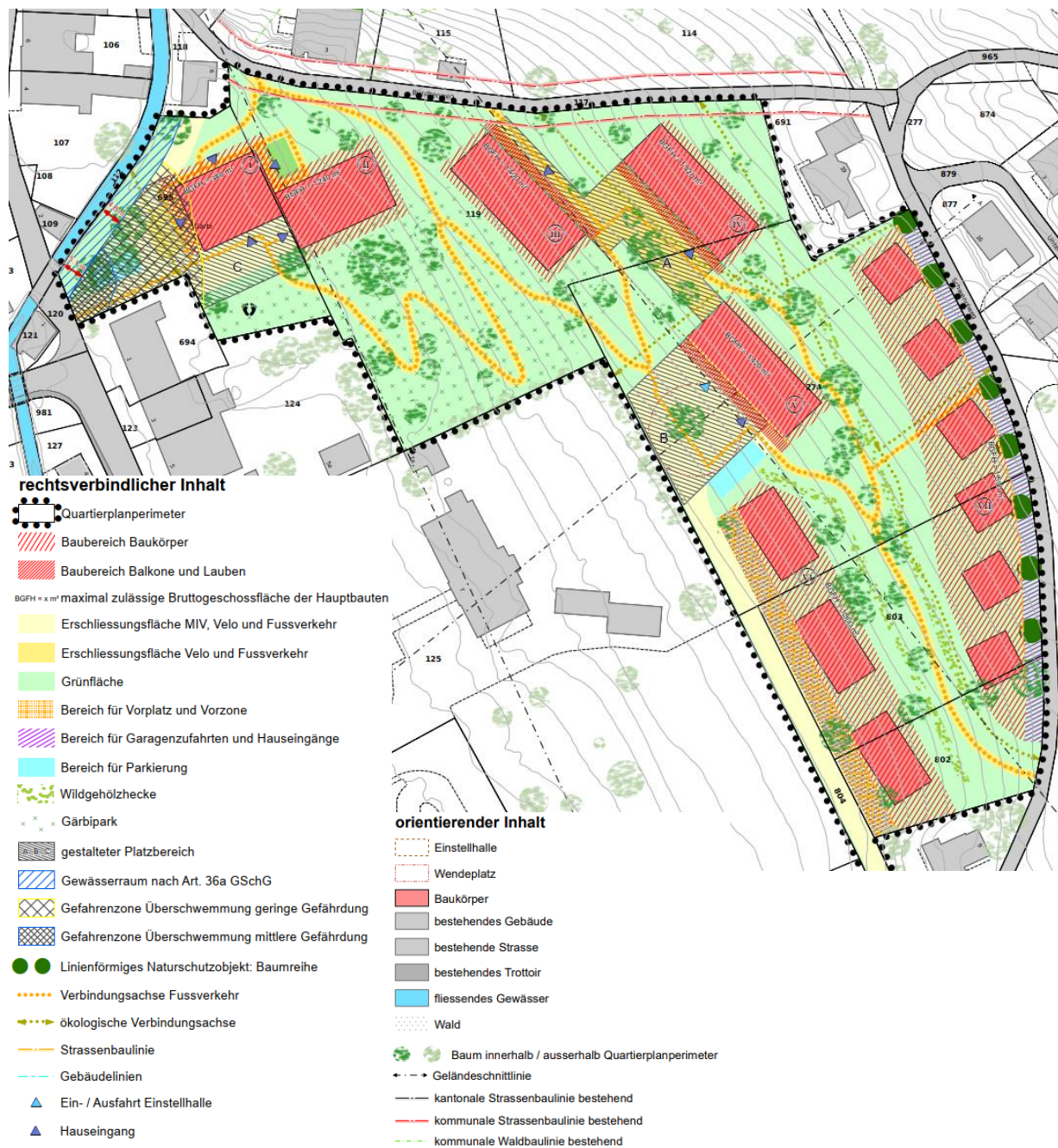
Abb. 12: Quartierplan Gärbi Bebauung / Erschliessung / Freiräume (Quelle: Jermann AG 2022)
